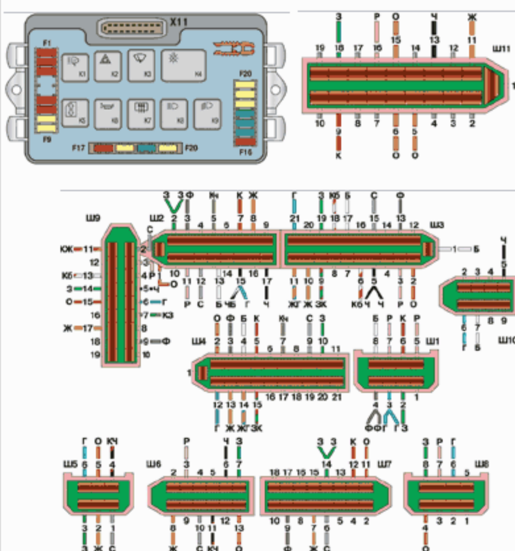
Рис. 7.2. Расположение реле и предохранителей в монтажном блоке 367.3722 (2114-3722): K1 – реле очистителей фар (в блоке 367.3722 отсутствует); K2 – реле-прерыватель указателей поворота и аварийной сигнализации; K3 – реле очистки ветрового стекла; K4 – реле контроля исправности ламп (в блоке 367.3722 отсутствует); K5 – реле включения стеклоподъемников (в блоке 367.3722 отсутствует); K6 – реле включения звуковых сигналов; K7 – реле включения обогрева заднего стекла; K8 – реле включения дальнего света; K9 – реле включения ближнего света; F1–F16 – плавкие предохранители; F17–F20 – запасные предохранители
