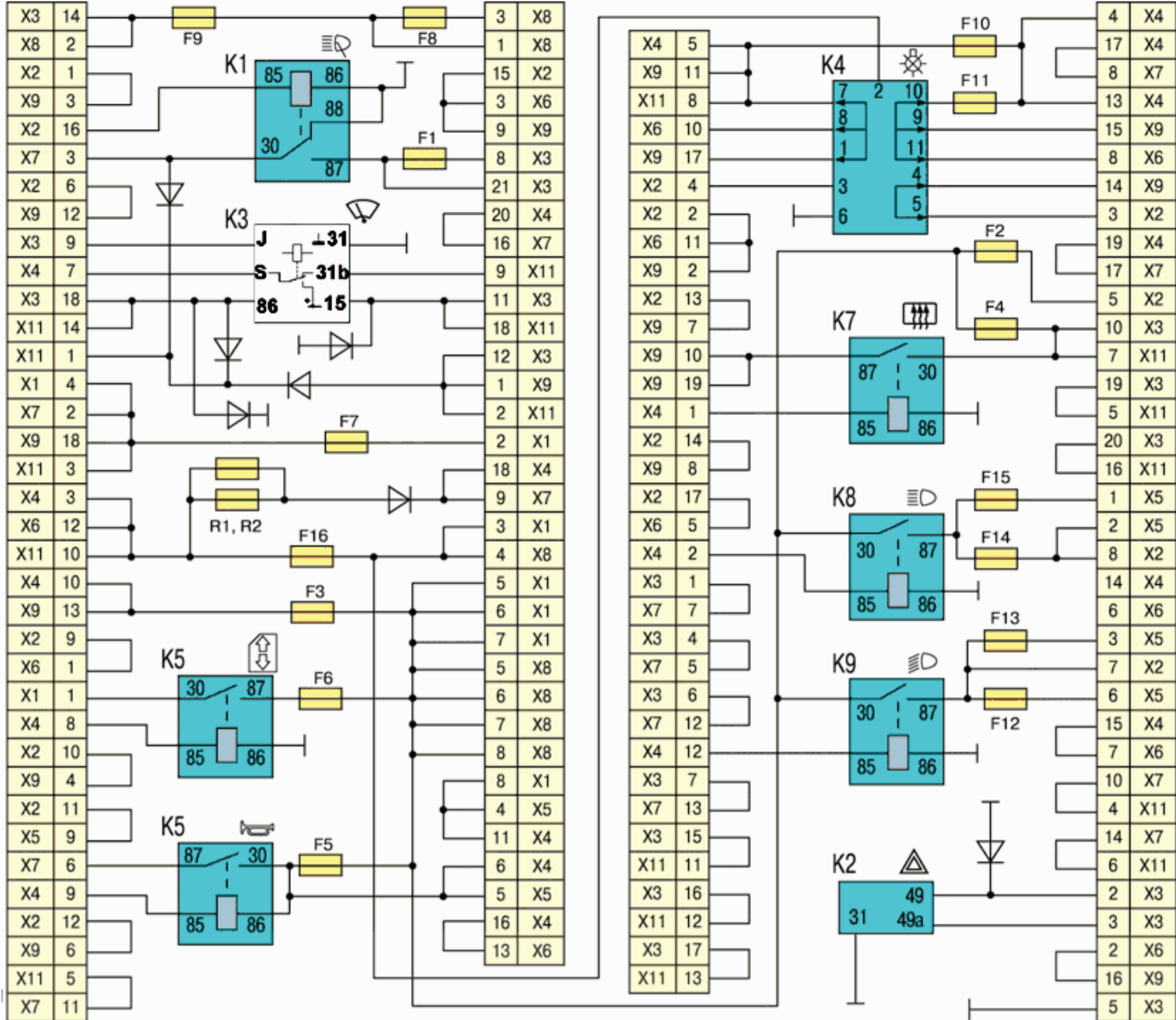
Рис. 7.2. Расположение реле и предохранителей в монтажном блоке 367.3722 (2114-3722): K1 – реле очистителей фар (в блоке 367.3722 отсутствует); K2 – реле-прерыватель указателей поворота и аварийной сигнализации; K3 – реле очистки ветрового стекла; K4 – реле контроля исправности ламп (в блоке 367.3722 отсутствует); K5 – реле включения стеклоподъемников (в блоке 367.3722 отсутствует); K6 – реле включения звуковых сигналов; K7 – реле включения обогрева заднего стекла; K8 – реле включения дальнего света; K9 – реле включения ближнего света; F1–F16 – плавкие предохранители; F17–F20 – запасные предохранители
